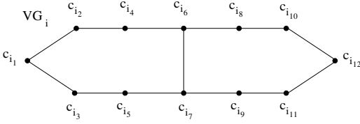
Fig. 1. A vertex gadget VG_i
